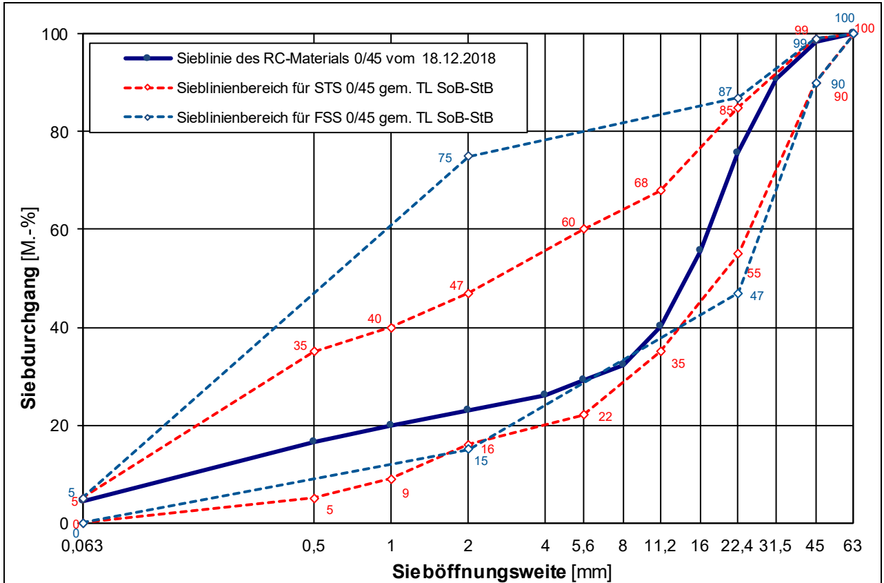
Korngrößenverteilung des untersuchten RC-Materials 0/45 mit Sieblinienbereich für Schottertrag- und Frostschutzschichten 0/45 mm gemäß TL SoB-StB /7/
