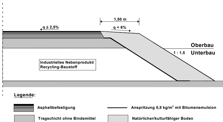
Bild 2: Damm, Abdeckung mit natürlichem/kulturfähigem Boden
