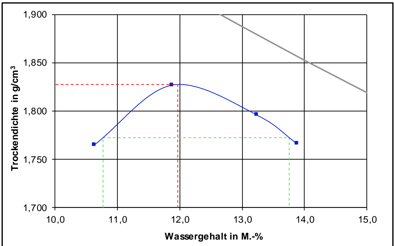
Proctorkurve des untersuchten RC-Materials 0/45 mm Juli 2019 (Prüfbericht Nr. F 19/07/1103)
