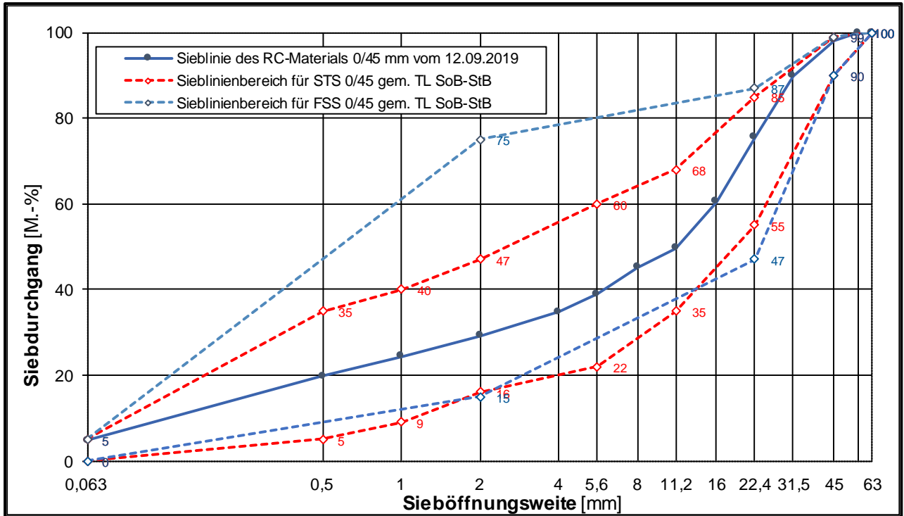
Korngrößenverteilung des untersuchten RC-Materials 0/45 mm mit Sieblinienbereich für Schottertrag- und Frostschutzschichten 0/45 mm gemäß TL SoB-StB /7/
