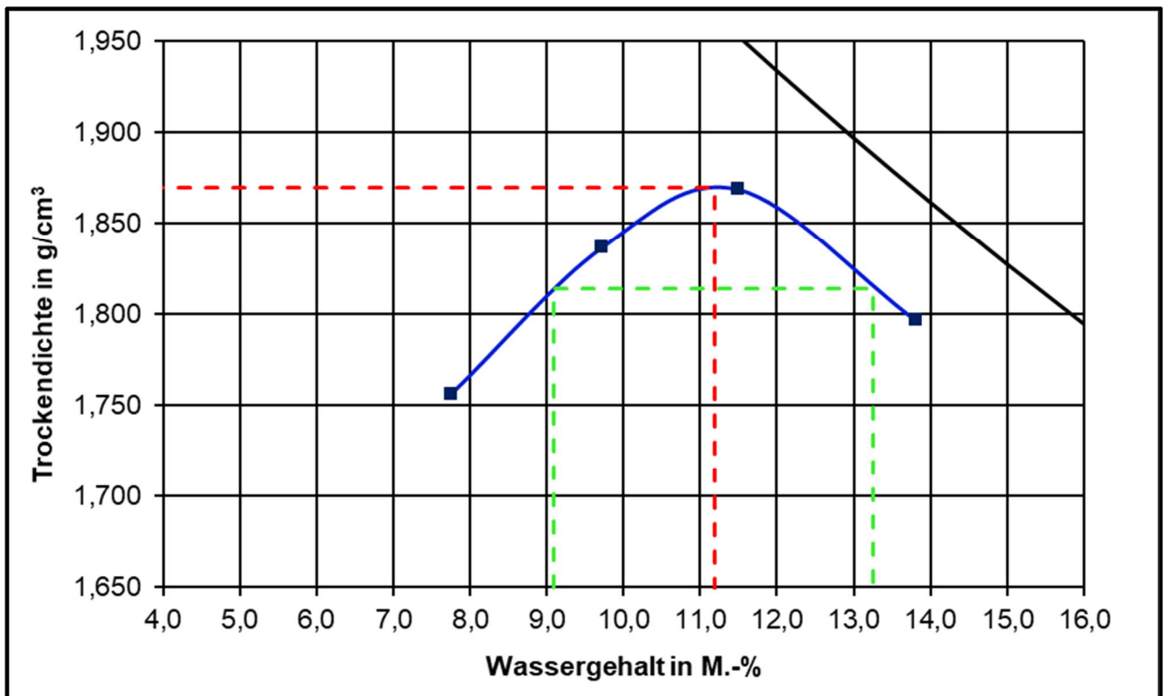
Proctorkurve des untersuchten RC-Materials 0/45 mm
