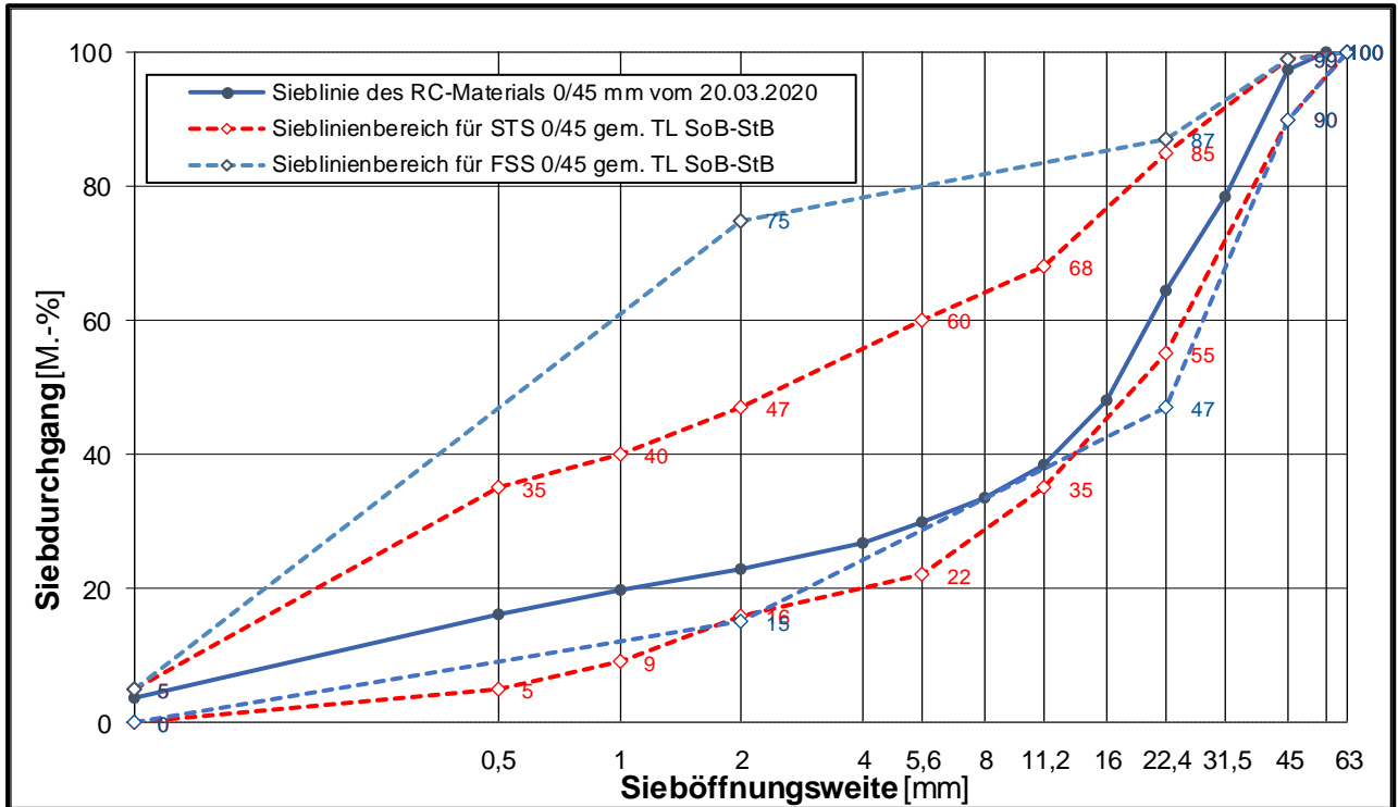
Korngrößenverteilung des untersuchten RC-Materials 0/45 mm mit Sieblinienbereich für Schottertrag- und Frostschuttschichten 0/45 mm gemäß TL SoB-StB /7/
