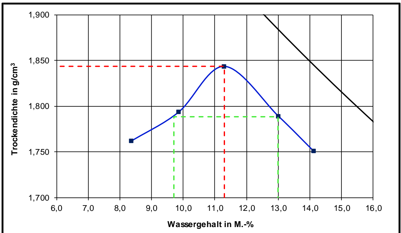
Proctorkurve des untersuchten RC-Materials 0/45 mm (aus Prüfbericht F 20/02/0119 – IV/2019)
