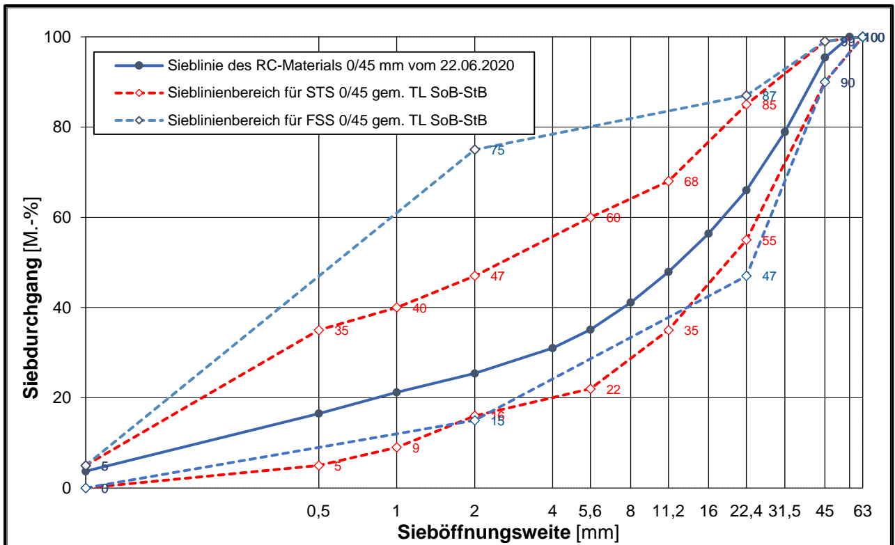
Korngrößenverteilung des untersuchten RC-Materials 0/45 mm mit Sieblinienbereich für Schottertrag- und Frostschutzschichten 0/45 mm gemäß TL SoB-StB //
