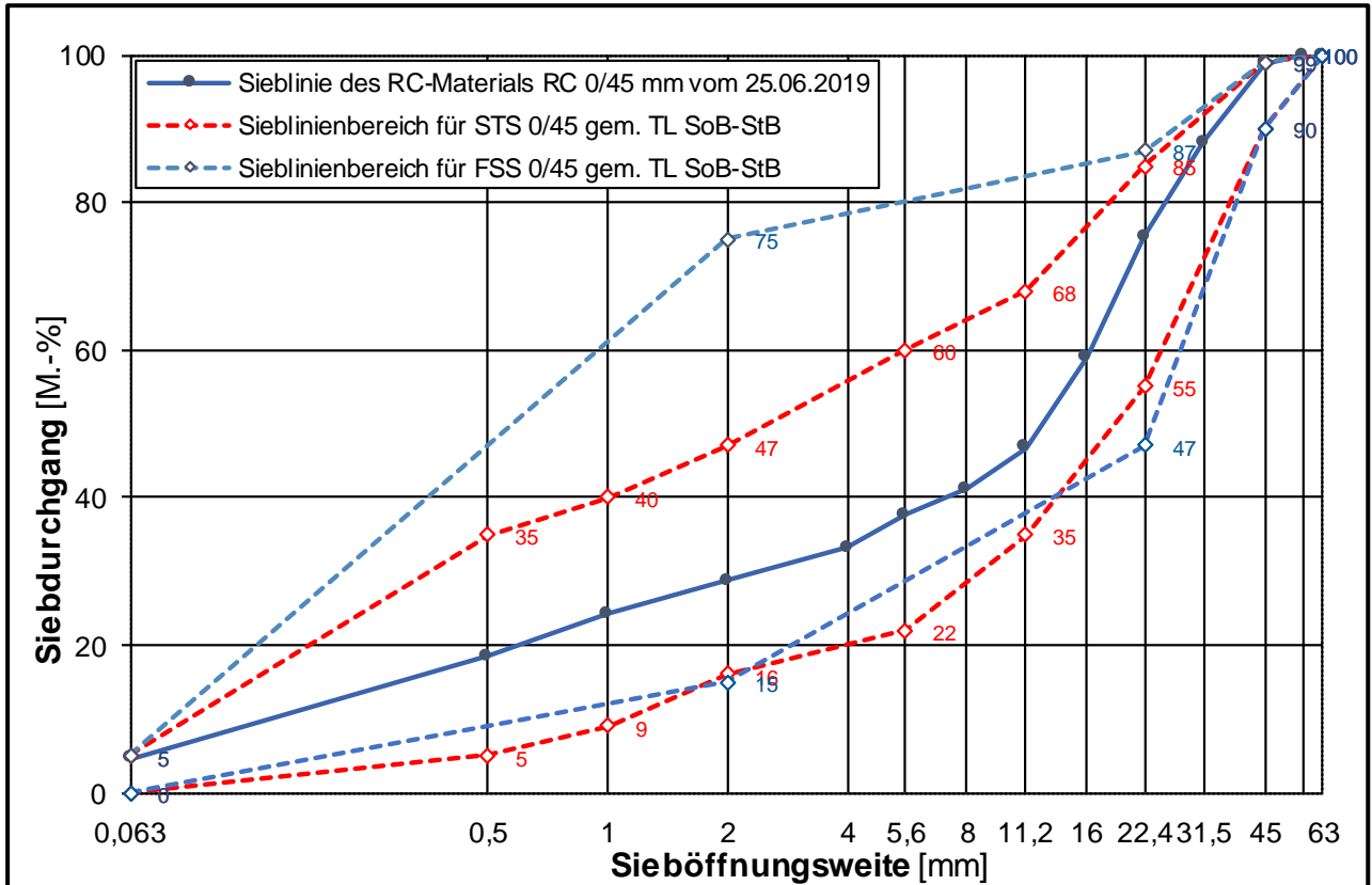
Korngrößenverteilung des untersuchten RC-Materials 0/45 mm mit Sieblinienbereich für Schottertrag- und Frostschutzschichten 0/45 mm gemäß TL SoB-StB 7/
